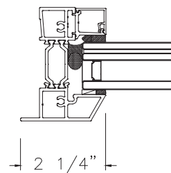
3C JAMB FIXED FLANGE
