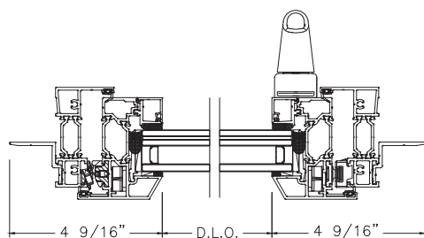
7B JAMB CASEMENT - FIN LEVER HANDLE
